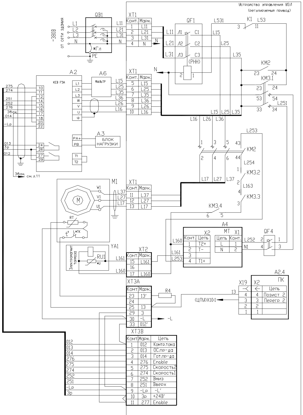
Рис. 2б (регулируемый привод с асинхронным двигателем)
