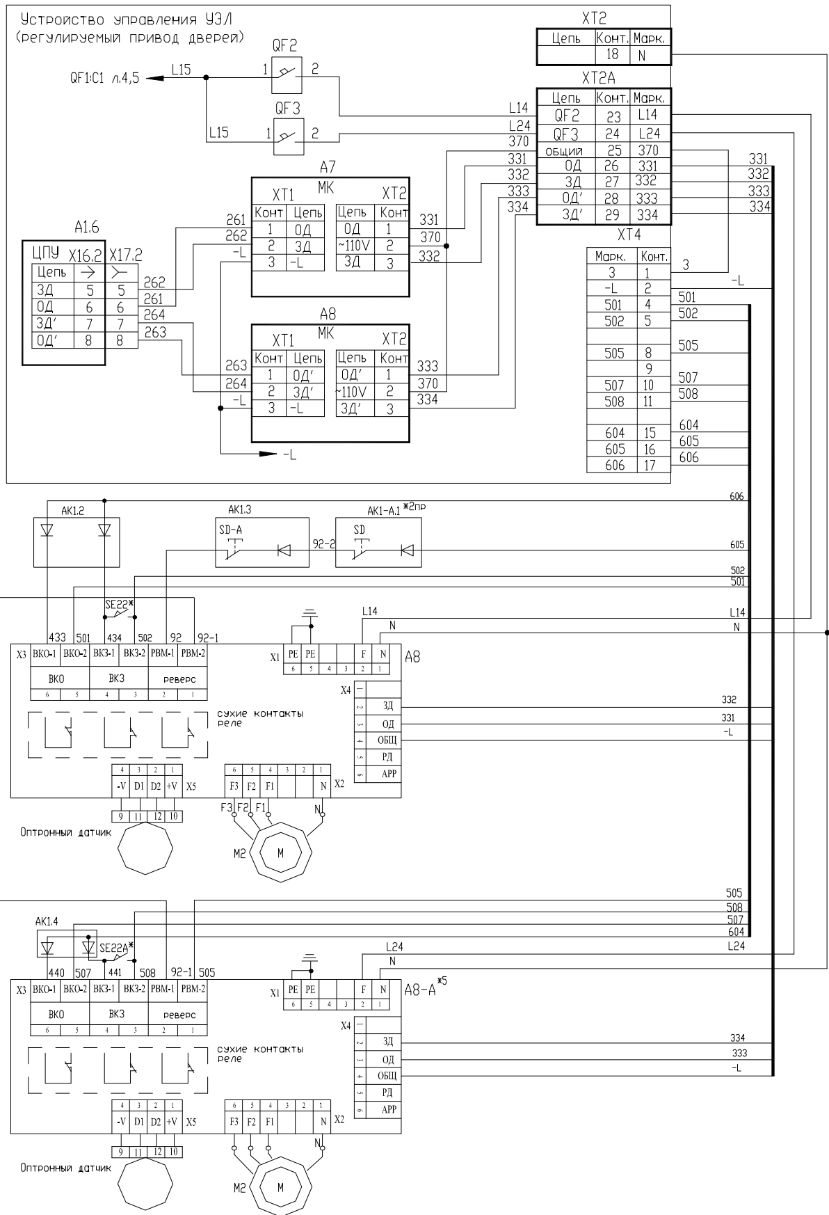
Рис.8 Схема управления приводом дверей
