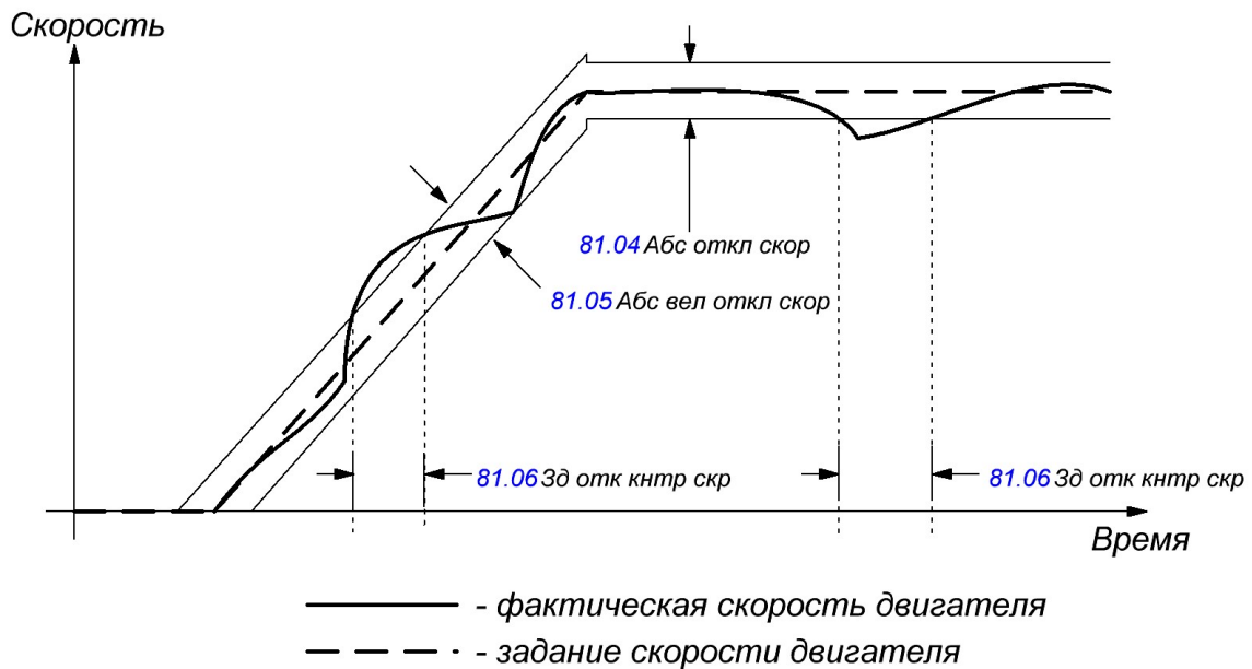
Рисунок 10.1 – Работа функции контроля скорости
